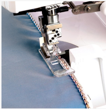
Pied transparent pour pose de perles
