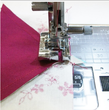
Pied patchwork pour couture ¼ de pouce sans guide (O)
