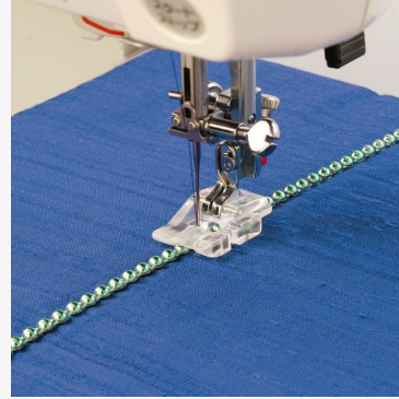
Pied pour pose de perles et de mèches de 2 et 4 mm
