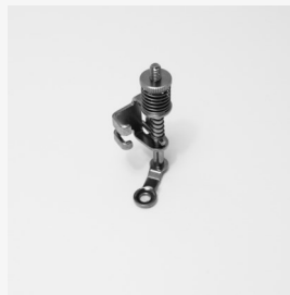
Pied pour quilting en piqué libre
