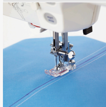
Pied transparent ¼ de pouce pour points droits (OM)
